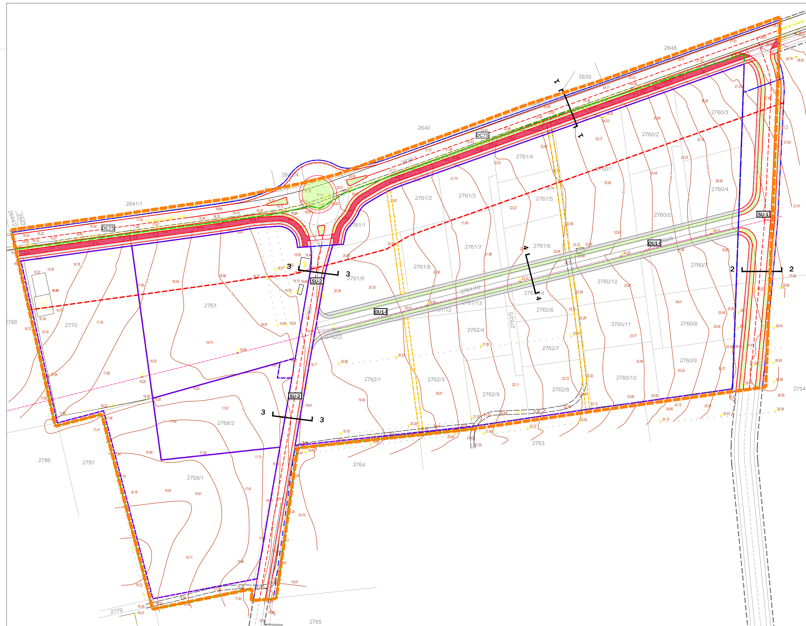
KARAKTERISTIČNI PRESJEKI PROMETNICA PRESJEK 1_1 JAVNA
