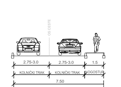
PRESJEK 3_3 JAVNA
