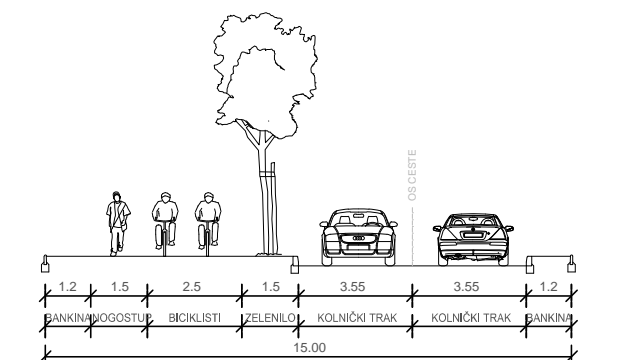
PRESJEK 2_2 JAVNA
