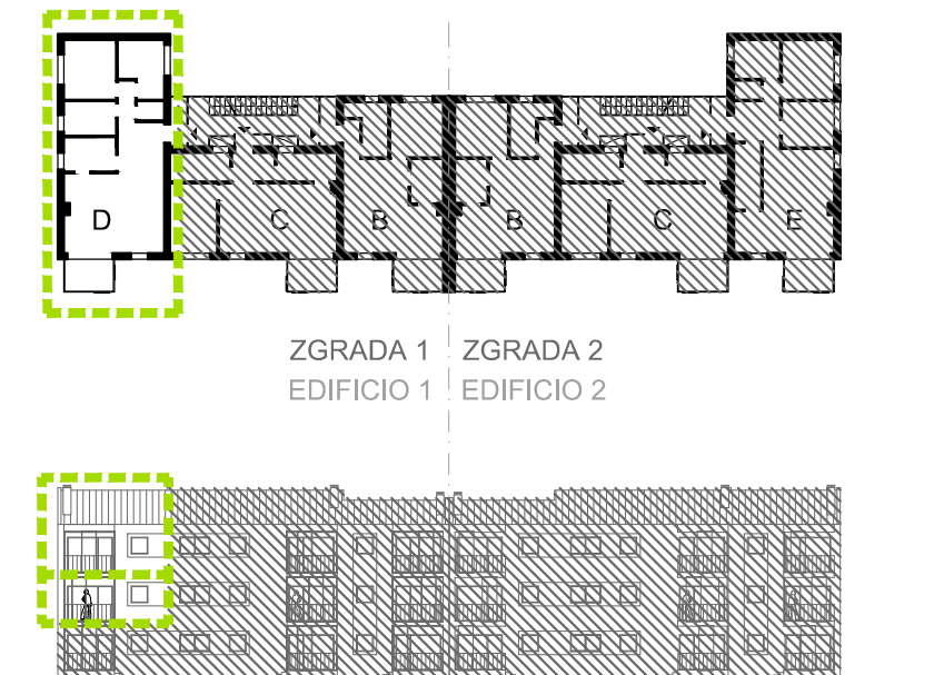
TLOCRT PRVOG KATA PIANTA DEL PRIMO PIANO
